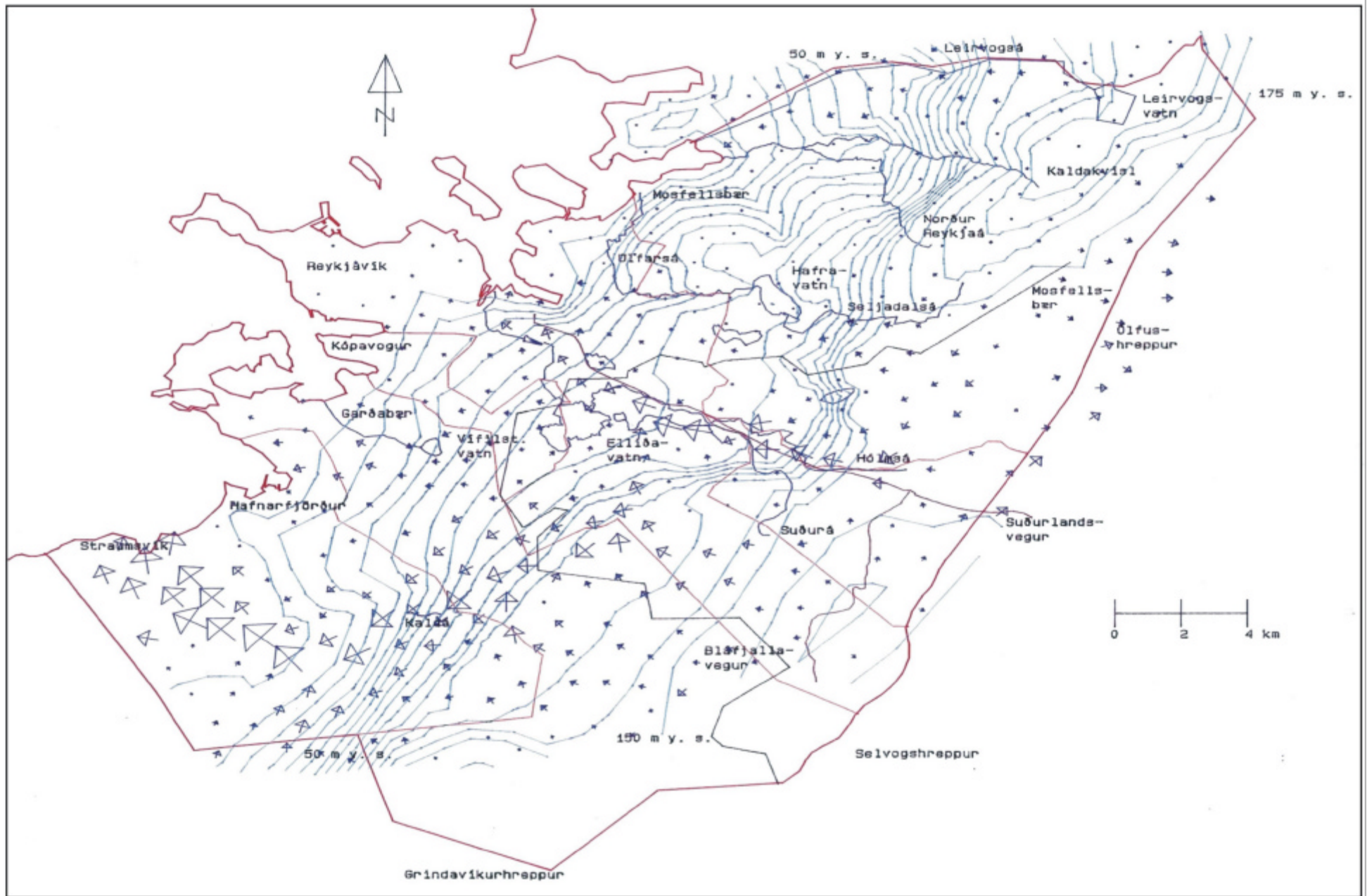
Mynd 9. Reiknuð grunnvatnshæð og grunnvatnsrennsli fyrir höfuðborgarsvæðið. Flæði (lítrar/sek/meter) er meira eftir því sem örvarnar eru lengri (Verkfræðistofan Vatnaskil, 1991).
